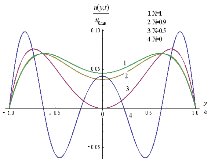
2.3-rasm. Yassi kanal kesimi bo‘yicha bo‘ylama tezlik tashkil etuvchisining tebranma oqimdagi ( \omega t = 0 , \alpha_0 = 3 bo‘lganda; 1 chiziq Nyuton suyuqligi 2-4 chiziqlar De = 1 bo‘lgandagi reologik murakkab suyuqlikning har xil konsentratsiyalaridagi) taqsimoti.
