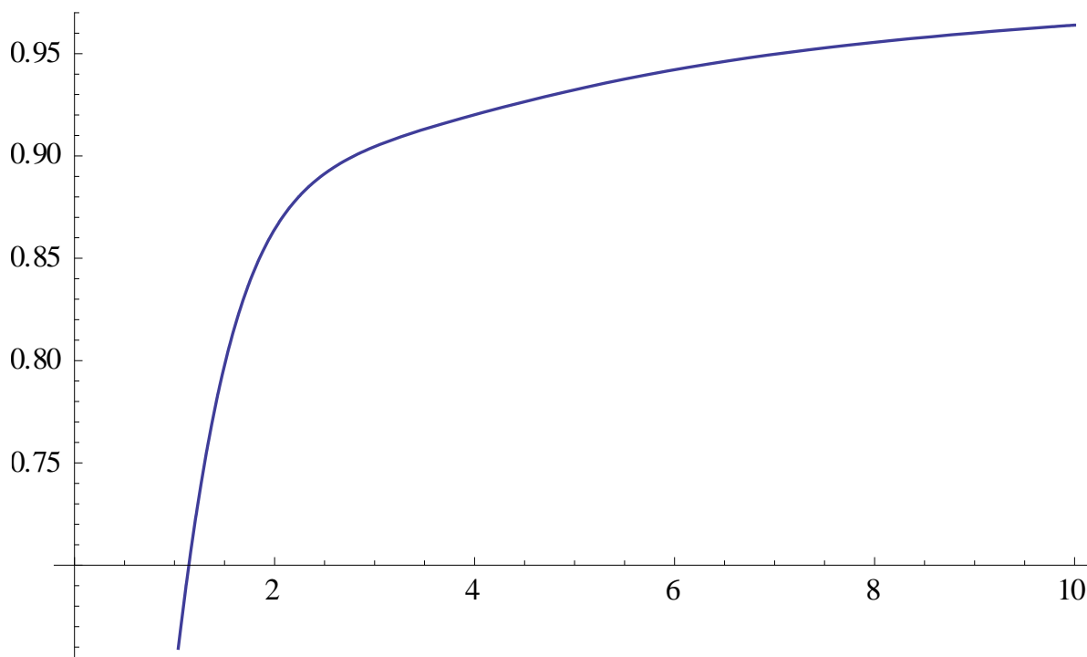
2.1-rasm. Nyuton suyuqligi pulsi oqimida bosim puls to‘lqini tarqalish tezligining, tebranish chastotasi parametriga bog‘liq o‘zgarishi
