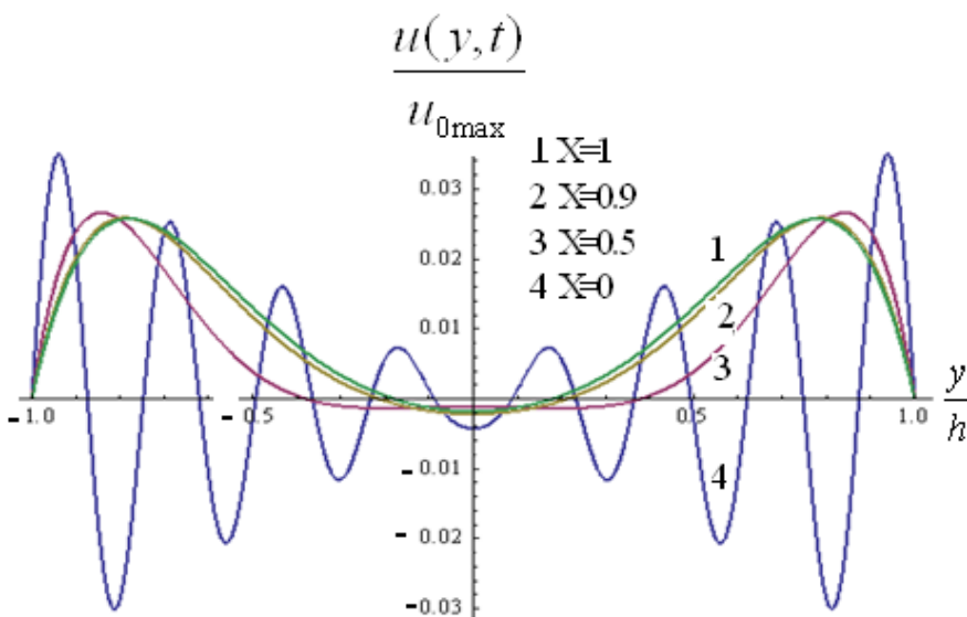
2.4-rasm. Yassi kanal kesimi bo‘yicha bo‘ylama tezlik tashkil etuvchisining tebranma oqimdagi ( \omega t = 0 , \alpha_0 = 5 bo‘lganda; 1 chiziq Nyuton suyuqligi, 2-4 chiziqlar De = 1 bo‘lgandagi reologik murakkab suyuqlikning har xil konsentratsiyalaridagi) taqsimoti.
